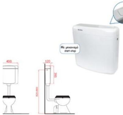
ΚΑΖΑΝΑΚΙ DALIA VIOSPIRAL ΥΨΗΛΗΣ ΠΙΕΣΕΩΣ
